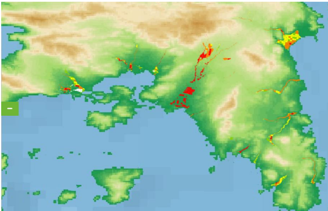
Εικόνα: Χάρτης Κινδύνου Πλημμύρας για T=1000
